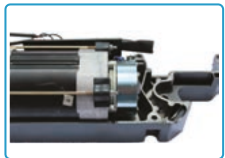
Freno solenoide de motor
