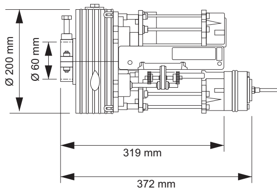
Dimensiones (mm) TIGER F260 / F360
